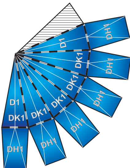
Spitze Bauteil D
