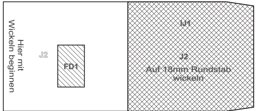
Innenverstärkung Bauteil J
